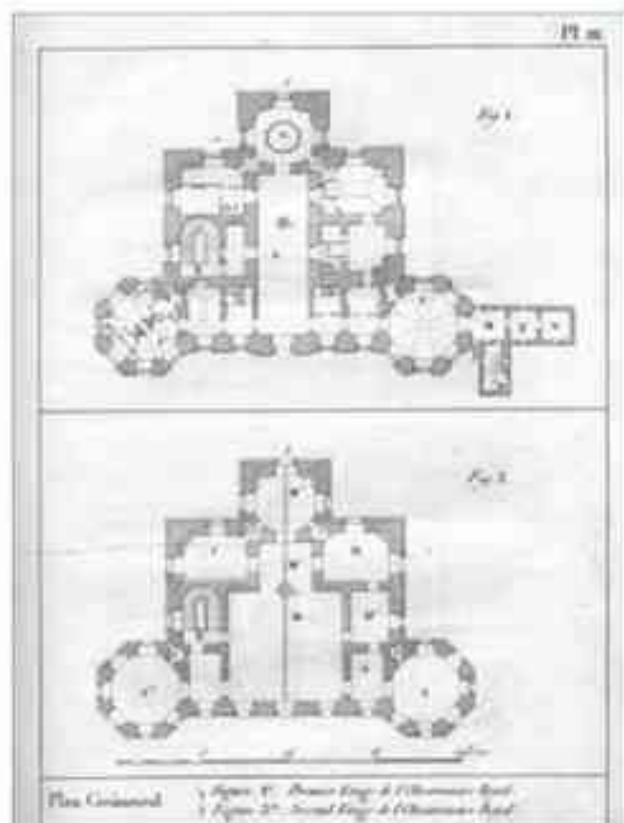
Figure 3. Plan des deux étages principaux de l'Observatoire à la fin du XVIII e siècle, avant les modifications de la saie de la méridienne. Le bâtiment était alors tel qu'il fut construit, sauf les salles d'observation MNON ajoutées à l'est en 1731. La méridienne du second étage, qui matérialise le méridien de Paris par une ligne de laiton inscrite dans le sol et permet de déterminer le midi vrai et la hauteur du Soleil à son passage au méridien, n'a été terminée qu'en 1729.
