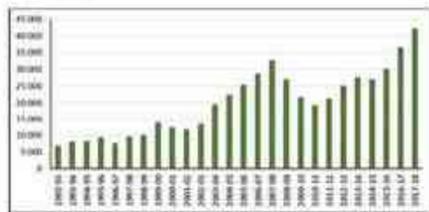
Fig 4 - Evolution du nombre de touristes transportés par navires et hélicoptère en Antarctique entre le début des années 1990 et aujourd'hui [Source : données IATO 2017 - http://www.ats.aq/documents/ATCM09/ATCM09_p153_rev1_e.doc ]
