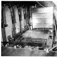
La machine à vapeur de la centrale électrique de la Sorbonne, construite en 1904, est la seule machine à vapeur de ce type qui reste en France. Elle est utilisée pour la production d'énergie électrique et pour la recherche scientifique.
